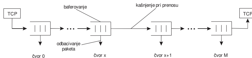
Slika 1. Kašnjenje/odbacivanje paketa u TCP konekciji Picture 1. Packet delay/dropp processes on a TCP connection
